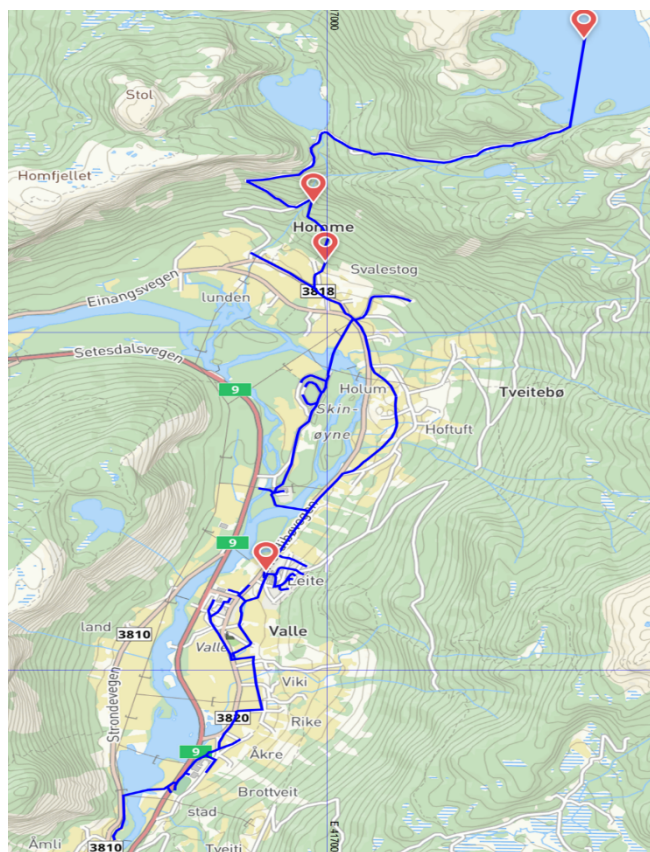
Kart over ledningsnett i Valle
